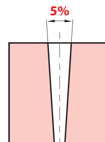
CONICITÉ 5% TAPER CONICIDAD 1:20 CONICITA'
