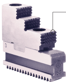
• Harte Aufsatzbacken FHB + FGB
